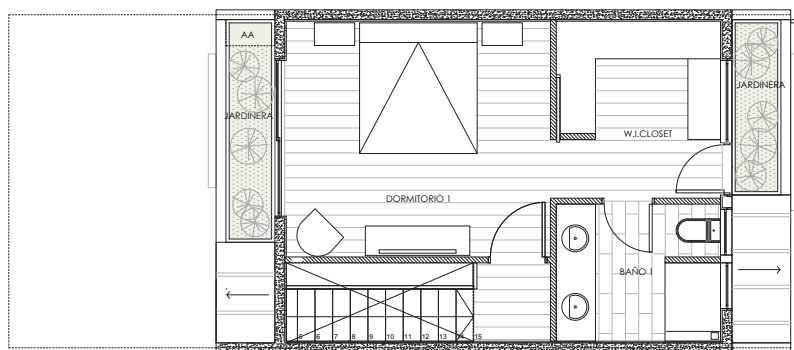
PLANTA 3º PISO
