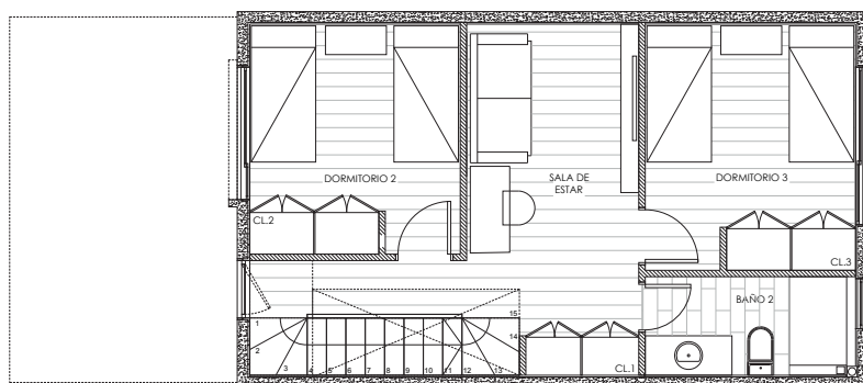
PLANTA 2º PISO
