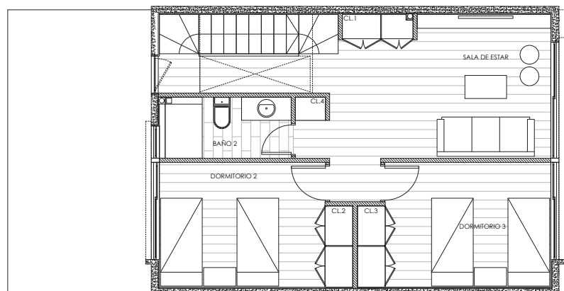
PLANTA 2° PISO
