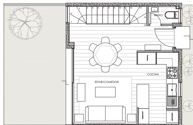
PLANTA 1° PISO
