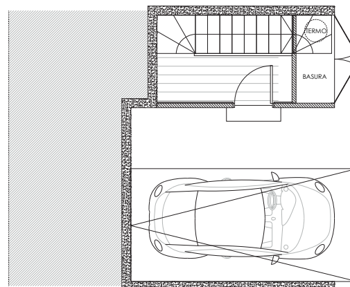
PLANTA SUBTERRÁNEO
