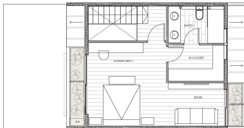
PLANTA 3° PISO
